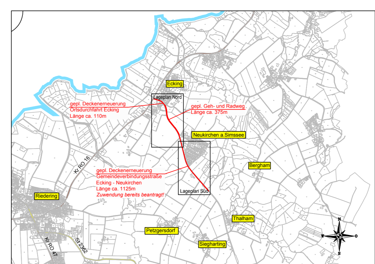
Übersichtslageplan, Maßstab = 1:25.000
